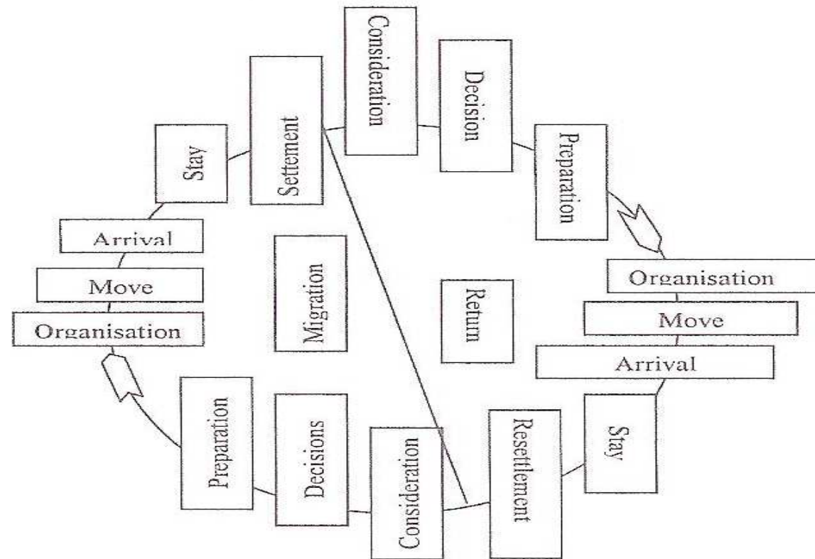
Grafik 1.1: Migrationsbahn („trajectory“)
